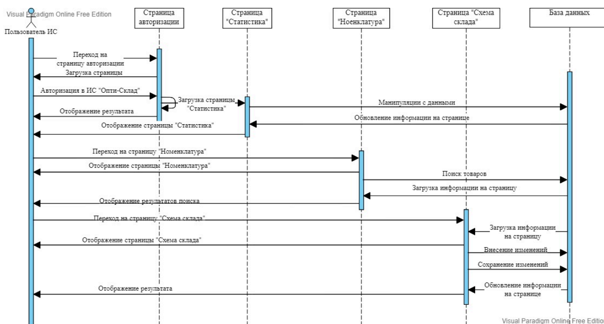
Рисунок 1 – Диаграмма последовательности действий пользователя
