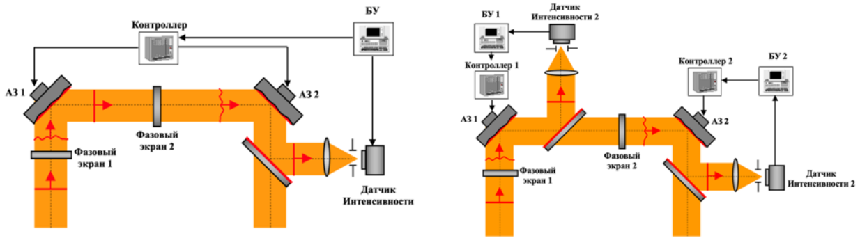
а) с общим блоком управления б) независимое управление двумя контурами Рисунок 1 – Схемы работы АОС с двумя адаптивными зеркалами
