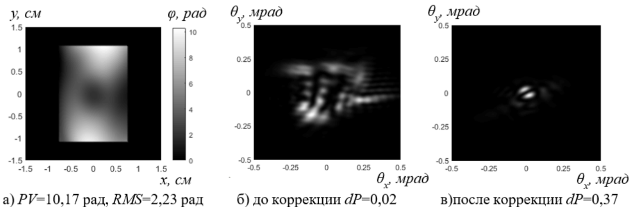
Рисунок 2 – Фазовый экран (а) и распределения интенсивности в дальней зоне до (б) и после (в) коррекции aberrаций
