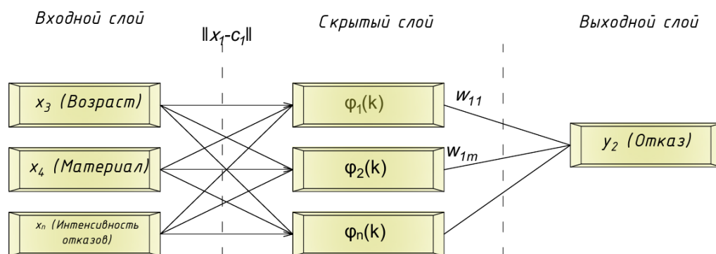
Рисунок 1 Структура нейронной сети обратного распространения
