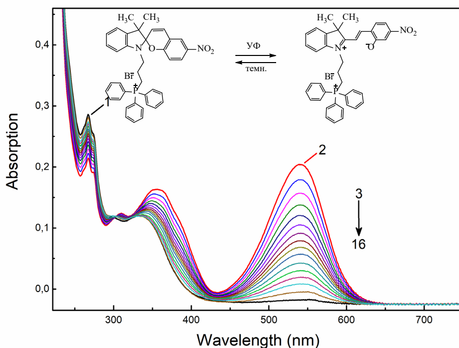
Рисунок 1. Спектр поглощения 3 в этаноле в спиропирановой (1) и мероцианиновой формах (2–16), измеренные до (1) и после УФ-облучения (2) через светофильтр УФС-1 и при обесцвечивании в темноте (3–16). C = 10^{-4} М,
