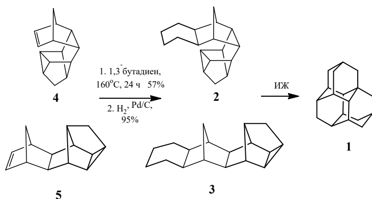
Схема 1. Синтез триамантана из углеводородов 4 и 5 в три стадии
