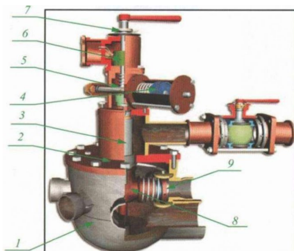
Рис.1 Переключатель скважин многоходовой
