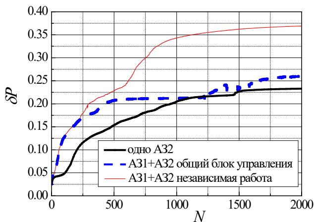
Рисунок 3 – Динамика работы СПГ алгоритма в АОС различных конфигураций
