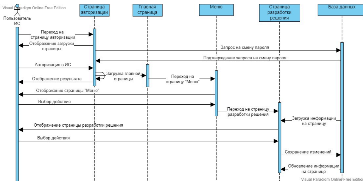
Рисунок 1 – Диаграмма последовательности действий пользователя
