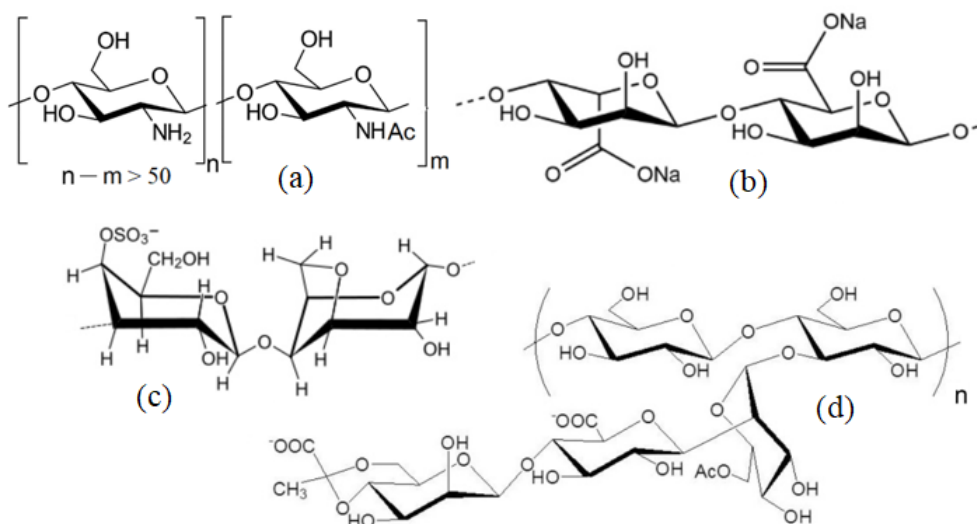
Рисунок 1. Формулы используемых полисахаридов: а – хитозан; б – альгинат натрия; с – к-каррагинан; д – ксантан (ксантановая камедь).
