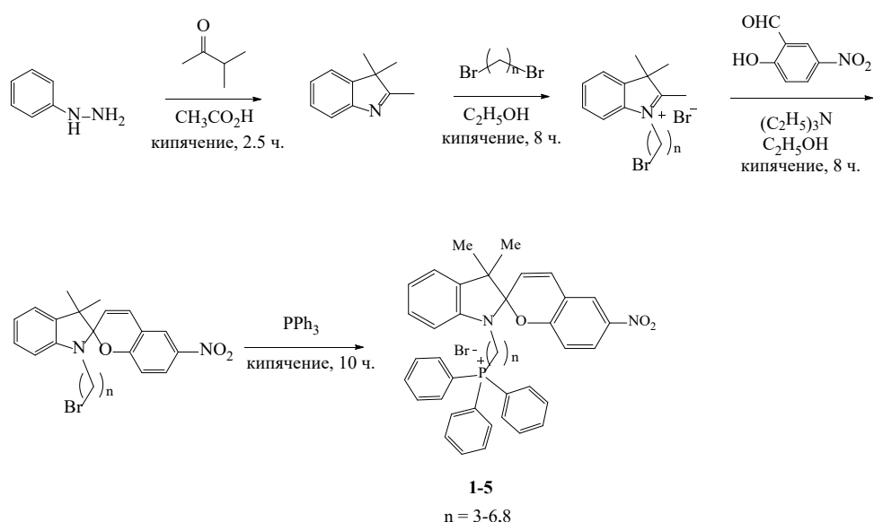
Схема 1. Синтез трифенилфосфониевых спиропирановых солей.
