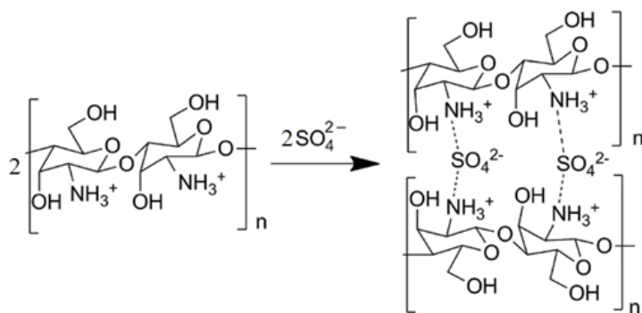
Рисунок 2. Сшивка протонированного хитозана (поликатионов хитозания) сульфат-анионами.
