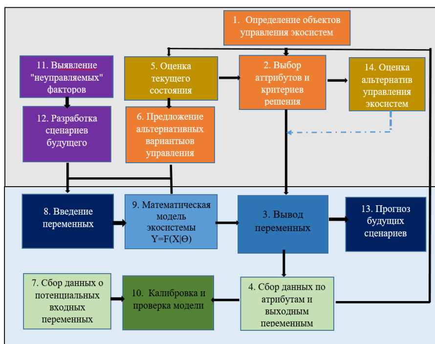
Рис. 2. Схематическое представление интеграции моделирования в процесс управления экосистемы
